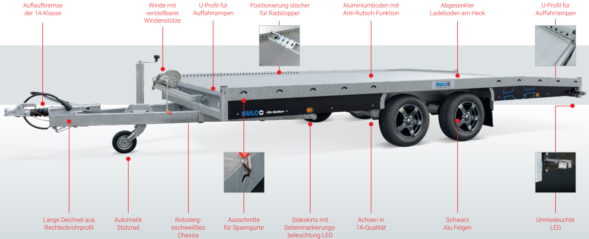
Extrem stabiles Fahrgestell mit optimaler Bodenunterstützung
